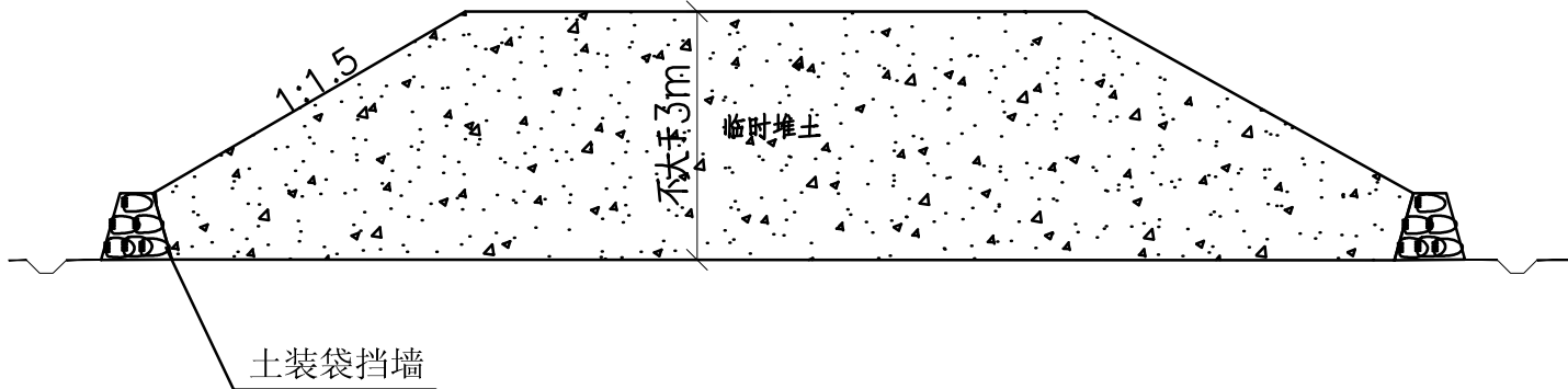
临时堆土场断面示意图
