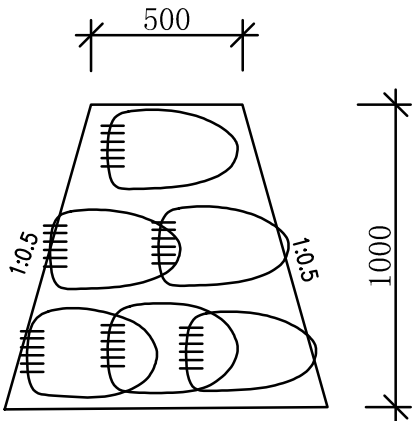
编织土袋挡墙断面图
