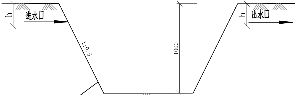
土质沉沙池纵断面图
